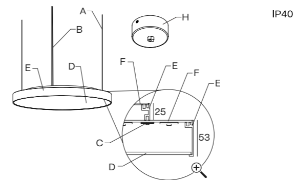
1. PENDANT - PENDANT UP LIGHT
