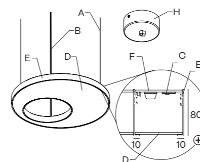
1. PENDANT - PENDANT UP LIGHT
