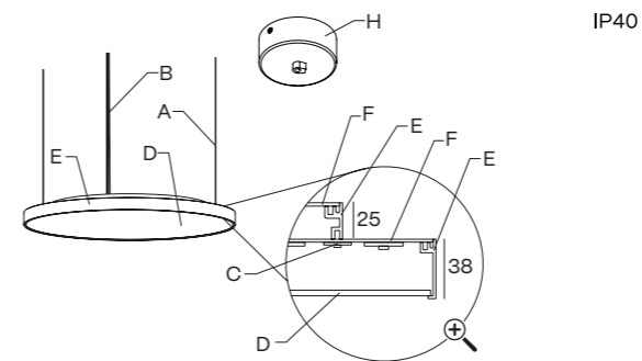
1. PENDANT - PENDANT UP LIGHT
